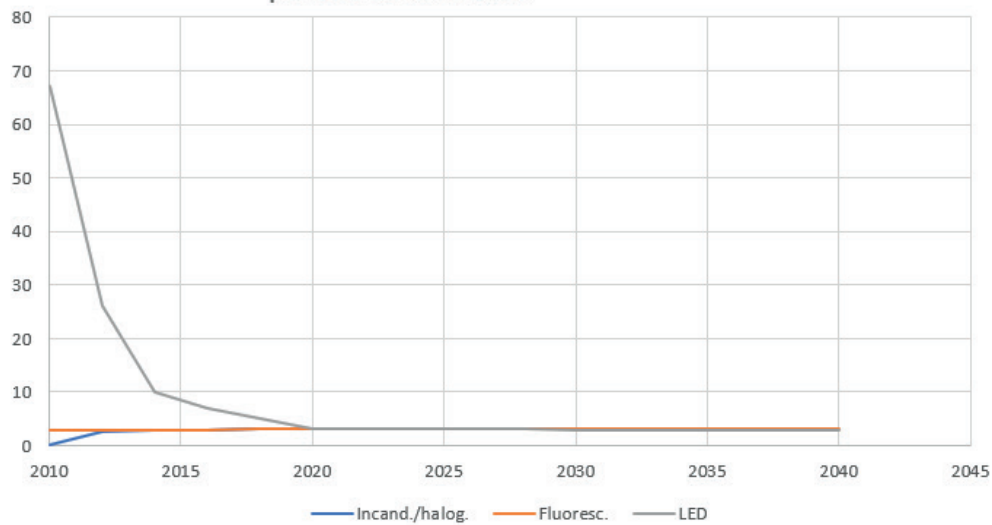
Coût relatif ($/lm) des technologies par source lumineuse
